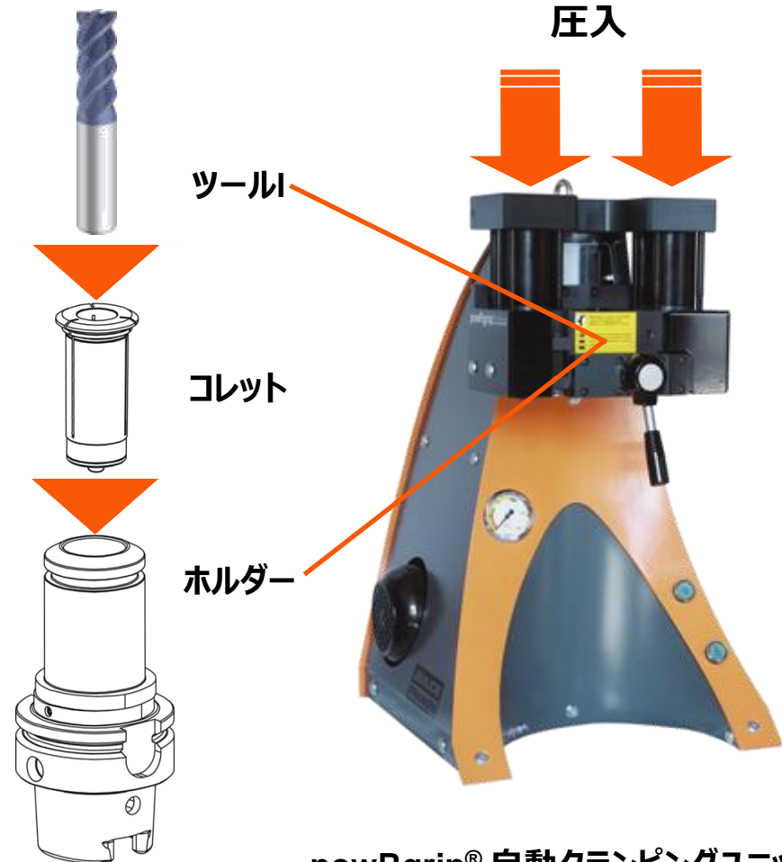
powRgrip® 自動クランピングユニット
